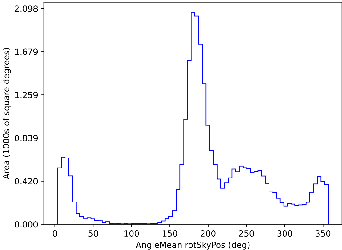
weather_cloudso2v3.4_10yrs All sky z band: AngleMean rotSkyPos
