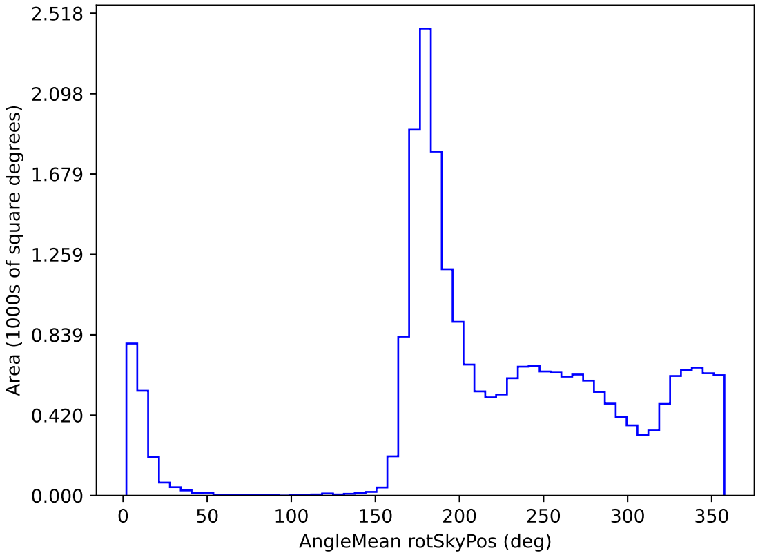
weather_cloudso2v3.4_10yrs All sky y band: AngleMean rotSkyPos
