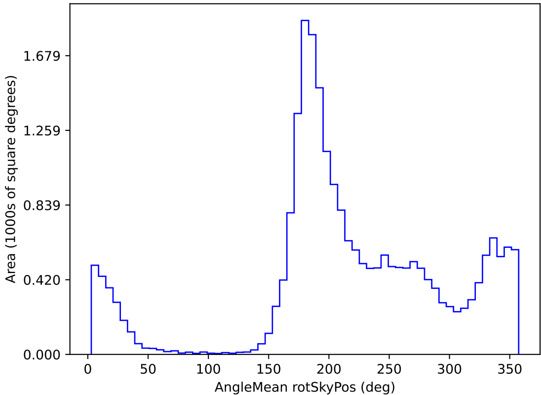
weather_cloudso2v3.4_10yrs All sky u band: AngleMean rotSkyPos
