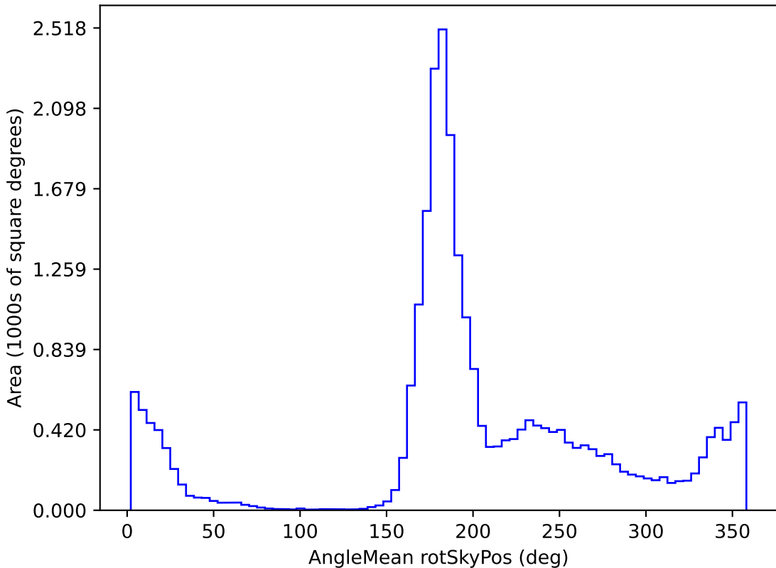
weather_cloudso2v3.4_10yrs All sky r band: AngleMean rotSkyPos
