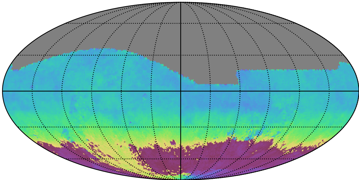
weather_cloudso2v3.4_10yrs All sky g band: AngleMean rotSkyPos
