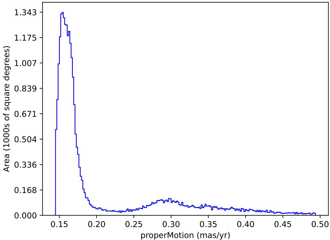
weather_cloudso2v3.4_10yrs : properMotion
