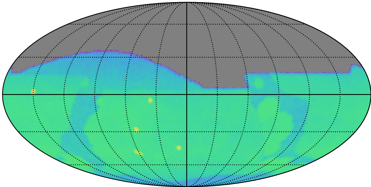
weather_cloudso2v3.4_10yrs g: CoaddM5
