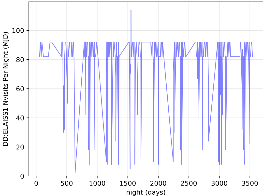
weather_cloudso2v3.4_10yrs all bands: DD:ELAISS1 Nvisits Per Night
