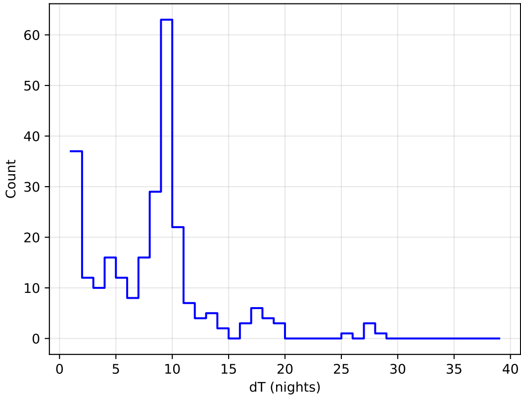
weather_cloudso2v3.4_10yrs all bands: DD:ELAISS1 Delta Nights Histogram
