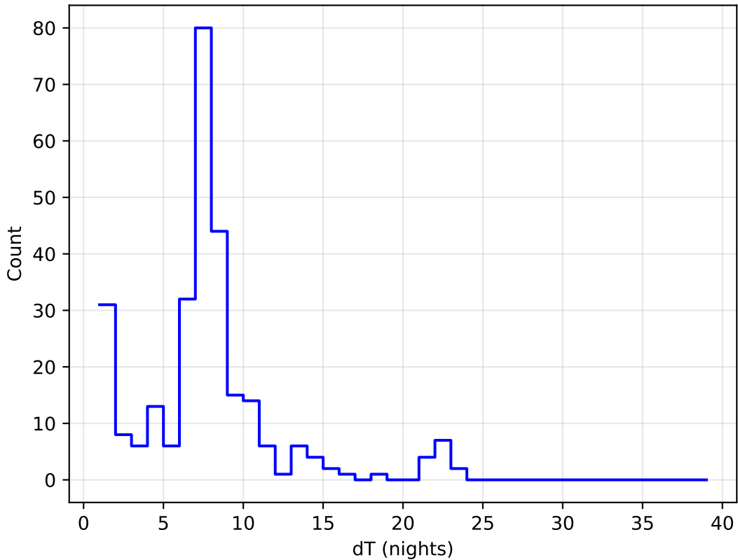
weather_cloudso2v3.4_10yrs all bands: DD:EDFS Delta Nights Histogram
