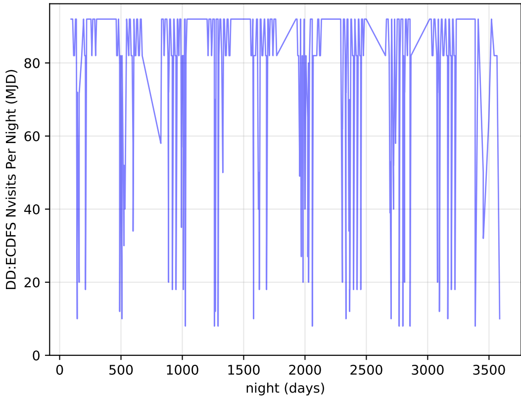
weather_cloudso2v3.4_10yrs all bands: DD:ECDFS Nvisits Per Night
