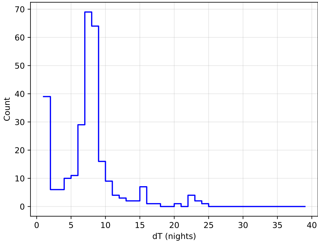
weather_cloudso2v3.4_10yrs all bands: DD:ECDFS Delta Nights Histogram
