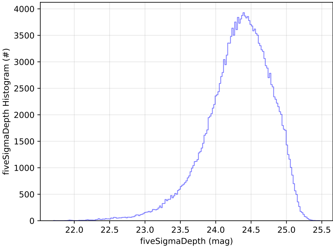
weather_cloudso20v3.4_10yrs g: fiveSigmaDepth Histogram
