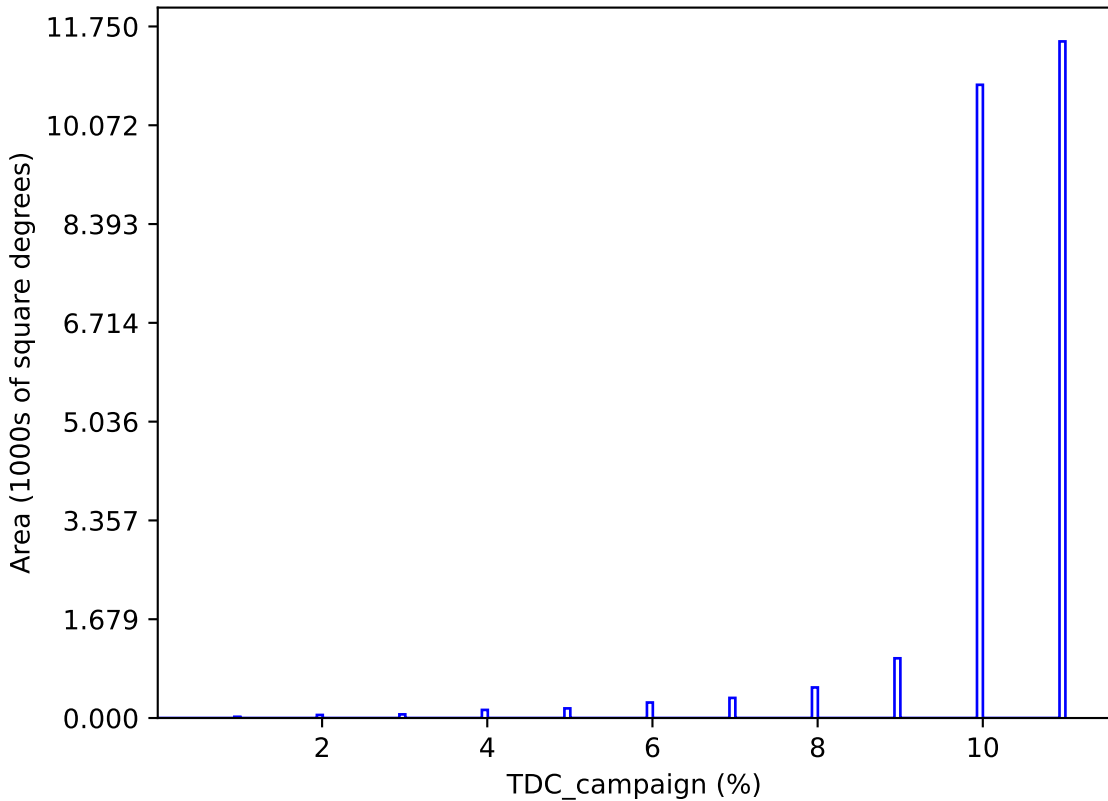
weather_cloudso20v3.4_10yrs : TDC_campaign
