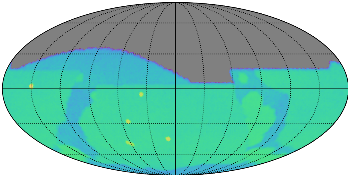
weather_cloudso20v3.4_10yrs g: SurfaceBrightLimit
