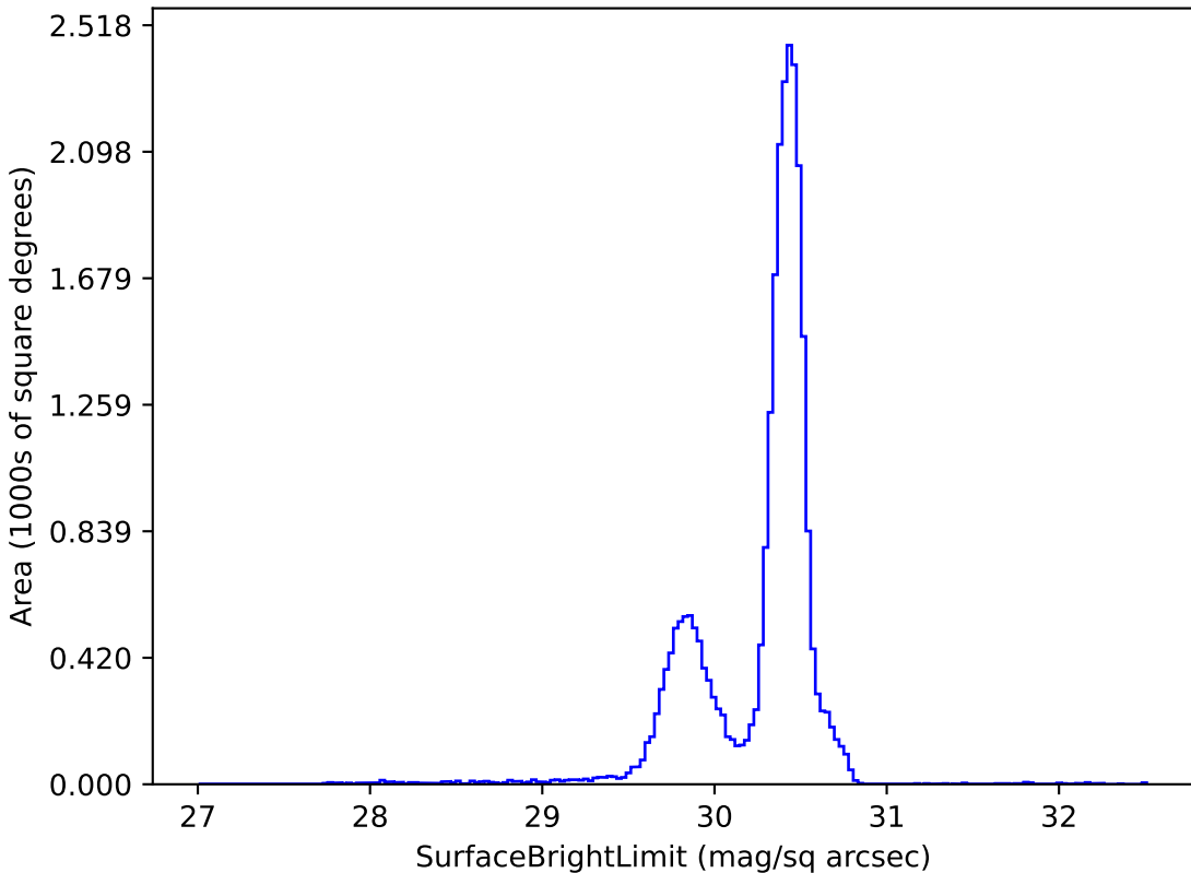
weather_cloudso20v3.4_10yrs g: SurfaceBrightLimit
