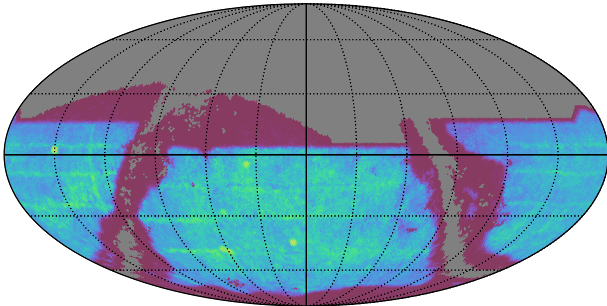
weather_cloudso20v3.4_10yrs : SNSLMetric
