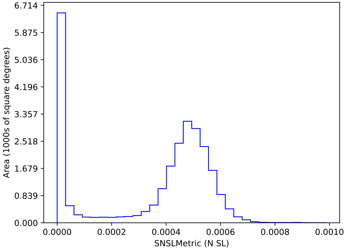
weather_cloudso20v3.4_10yrs : SNSLMetric
