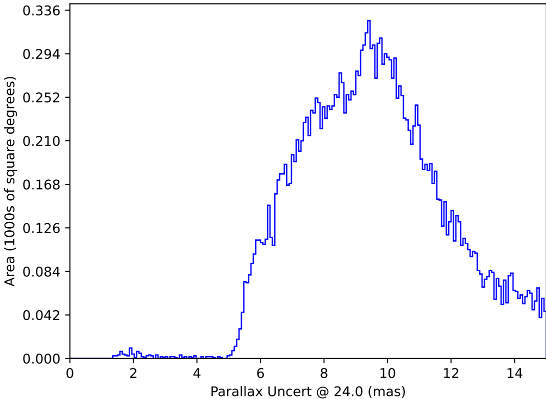
weather_cloudso20v3.4_10yrs : Parallax Uncert @ 24.0
