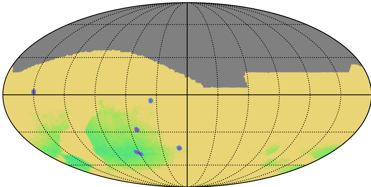
weather_cloudso20v3.4_10yrs : Parallax Uncert @ 22.4
