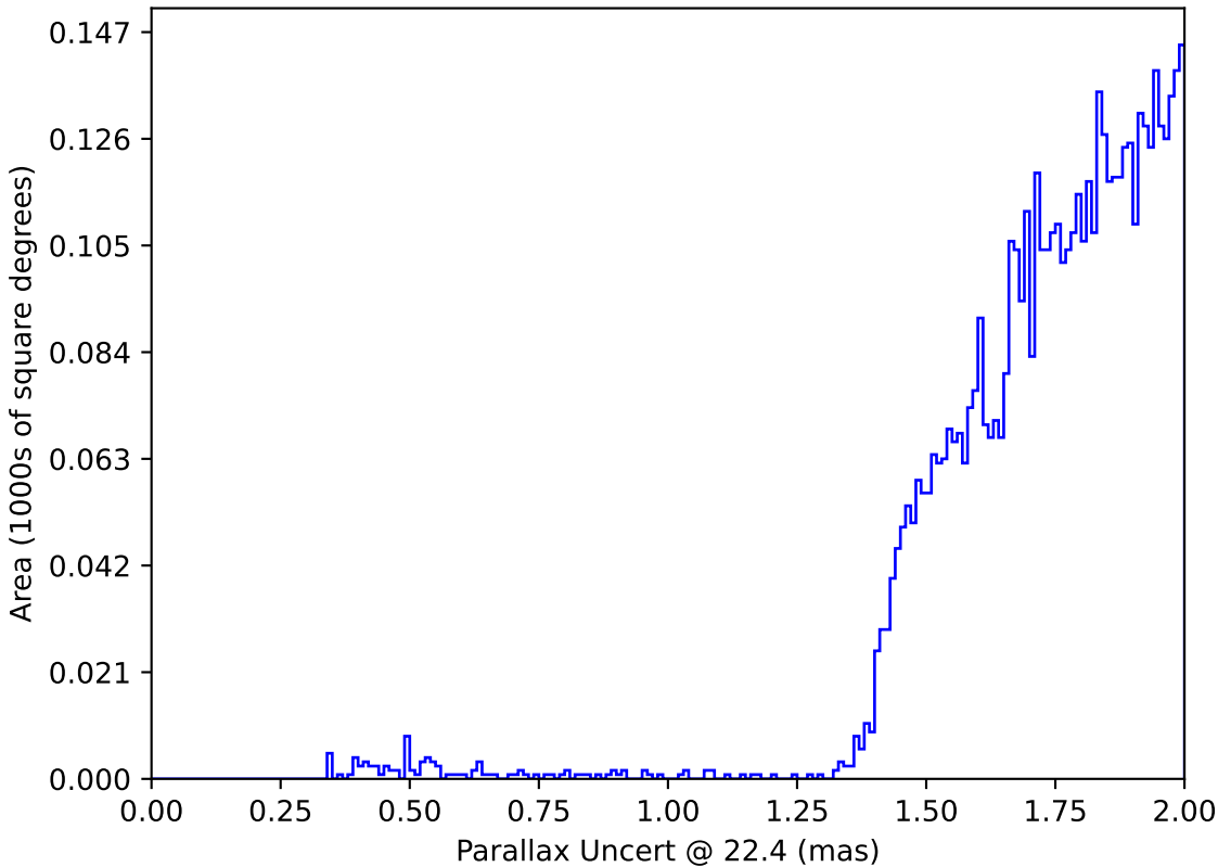
weather_cloudso20v3.4_10yrs : Parallax Uncert @ 22.4
