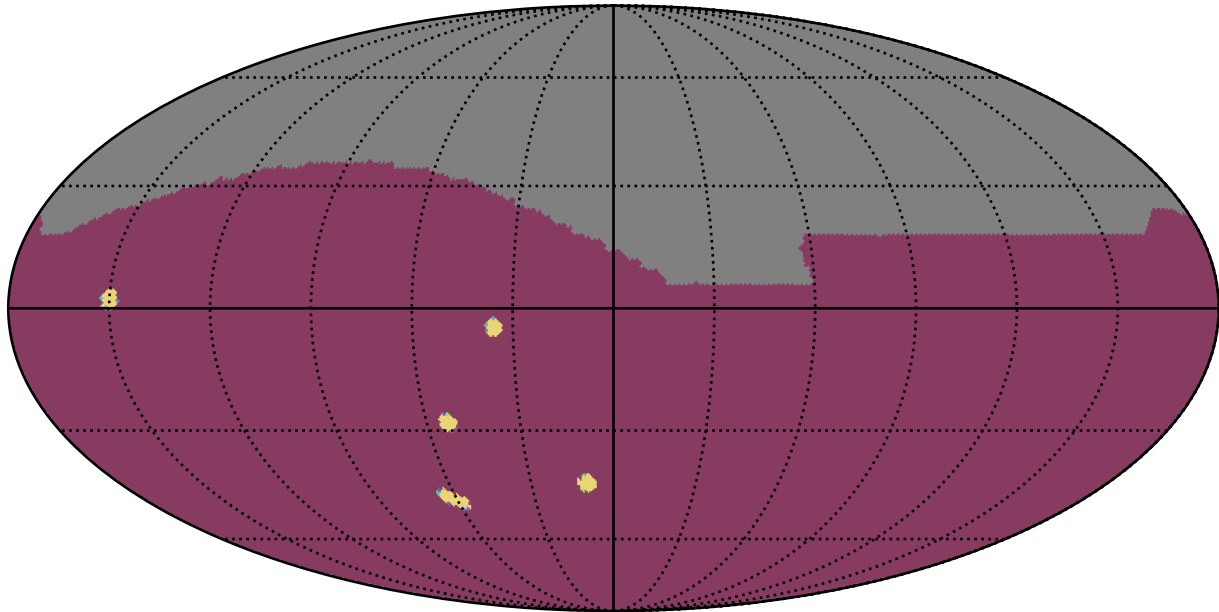
weather_cloudso20v3.4_10yrs : NumberOfQuickRevisits
