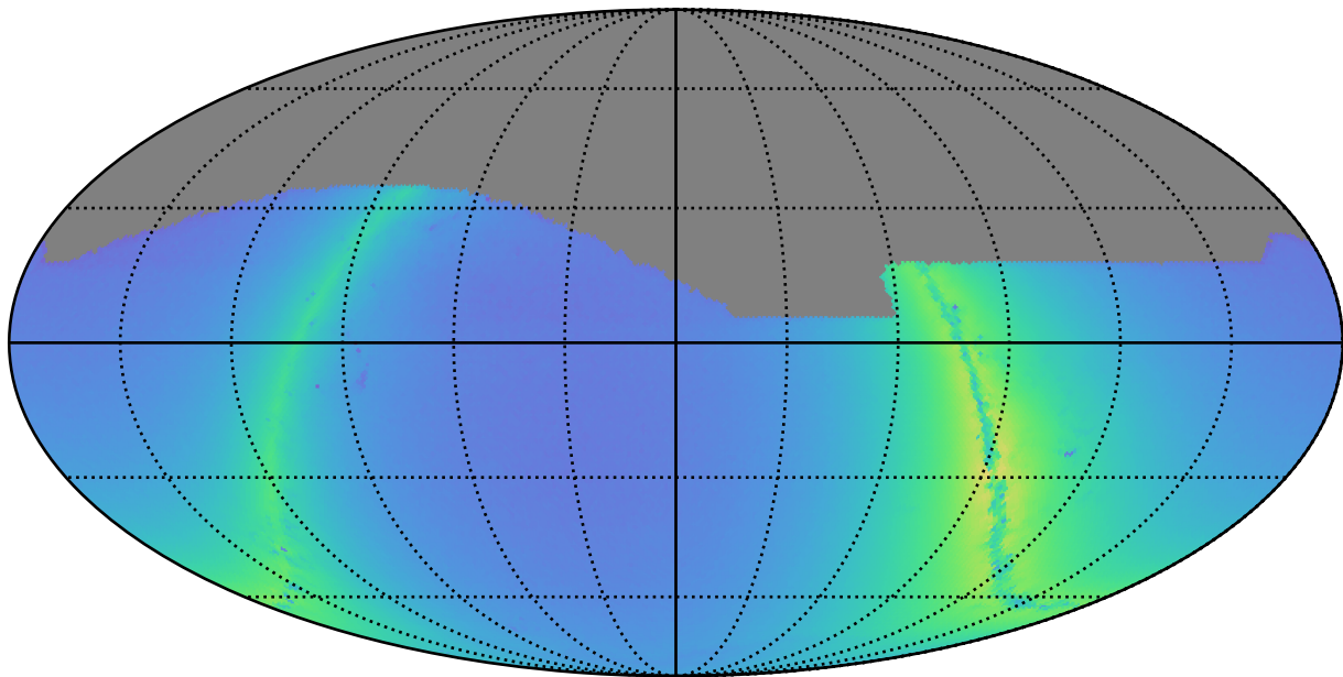
weather_cloudso20v3.4_10yrs z: Nstars_no_crowding
