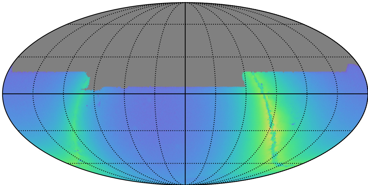
weather_cloudso20v3.4_10yrs y: Nstars_no_crowding
