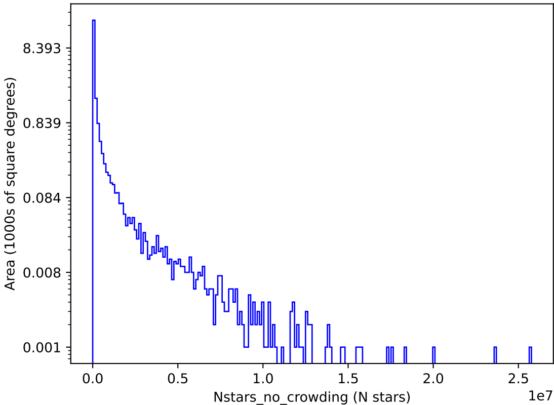
weather_cloudso20v3.4_10yrs y: Nstars_no_crowding
