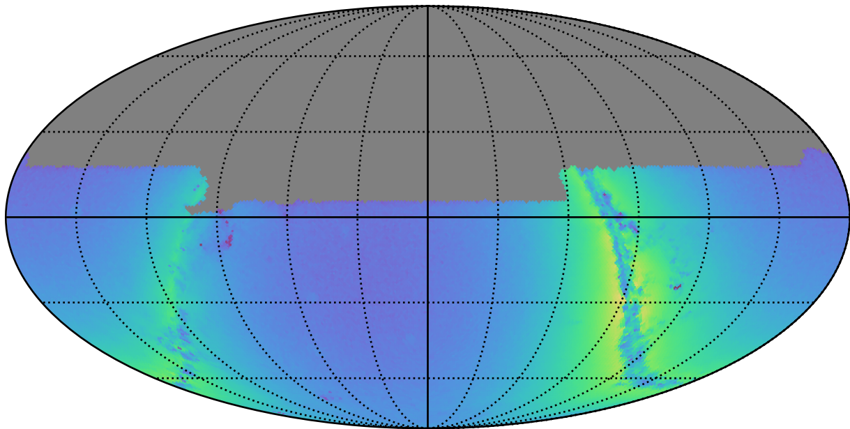
weather_cloudso20v3.4_10yrs u: Nstars_no_crowding
