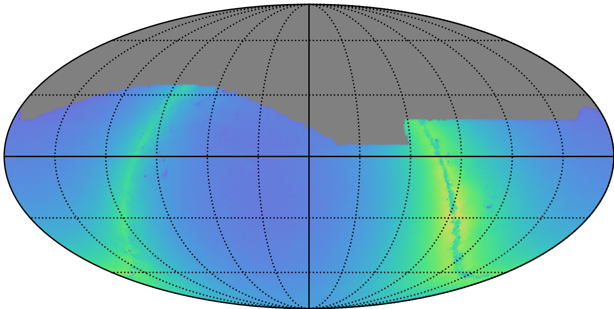
weather_cloudso20v3.4_10yrs r: Nstars_no_crowding
