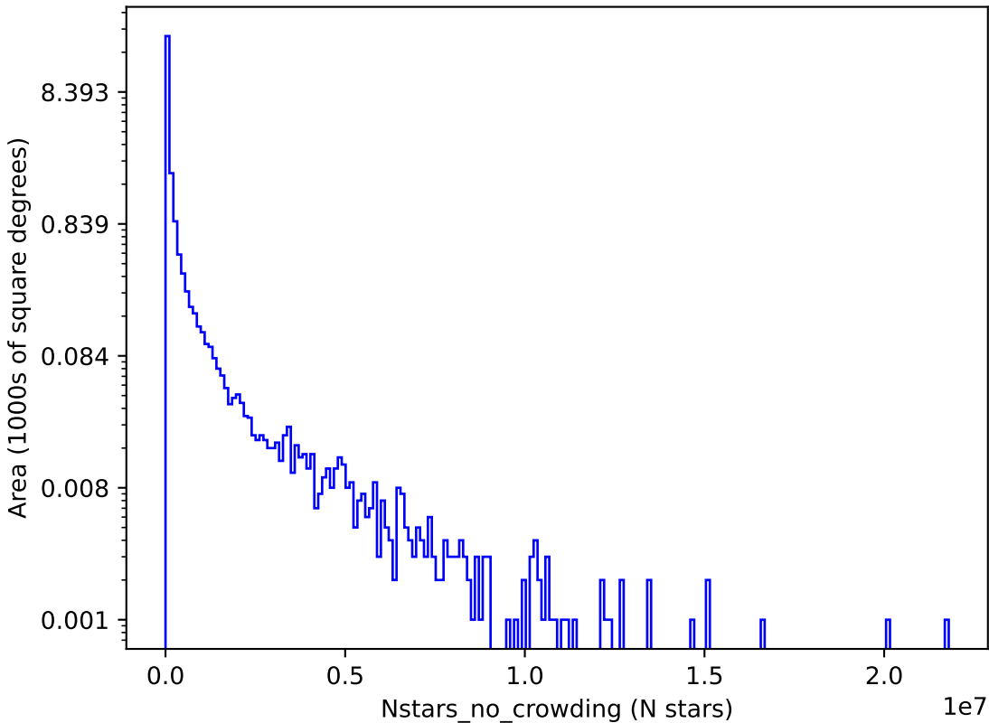
weather_cloudso20v3.4_10yrs r: Nstars_no_crowding
