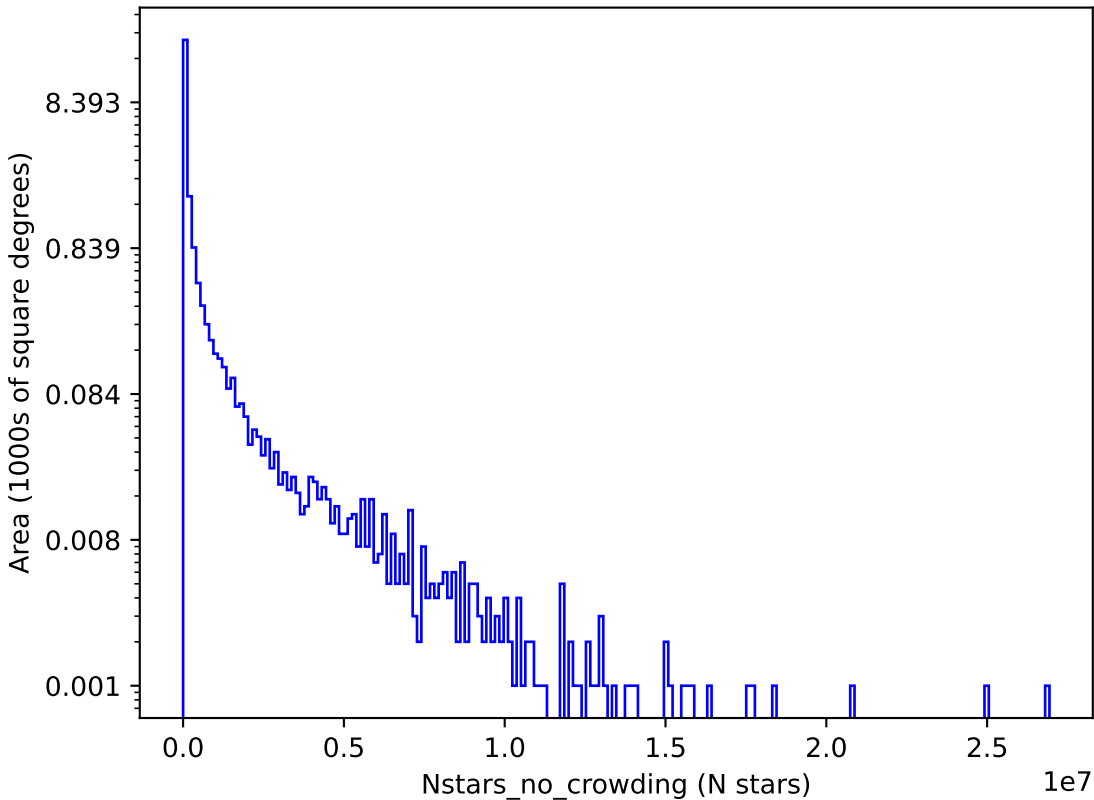
weather_cloudso20v3.4_10yrs i: Nstars_no_crowding
