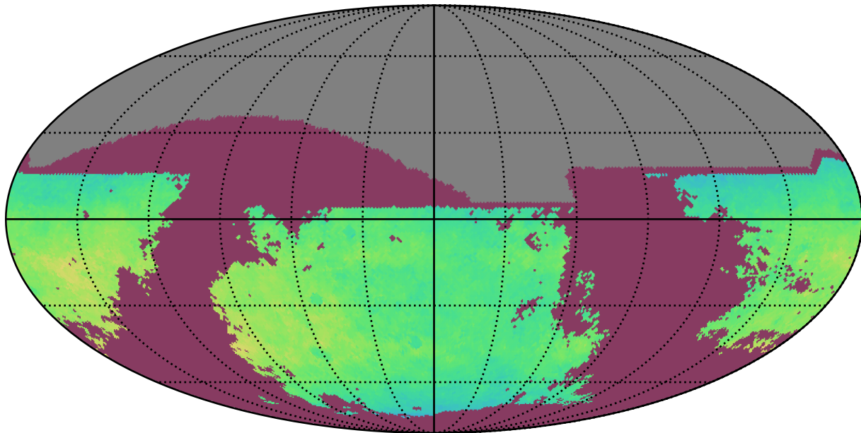
weather_cloudso20v3.4_10yrs i: NgalScale
