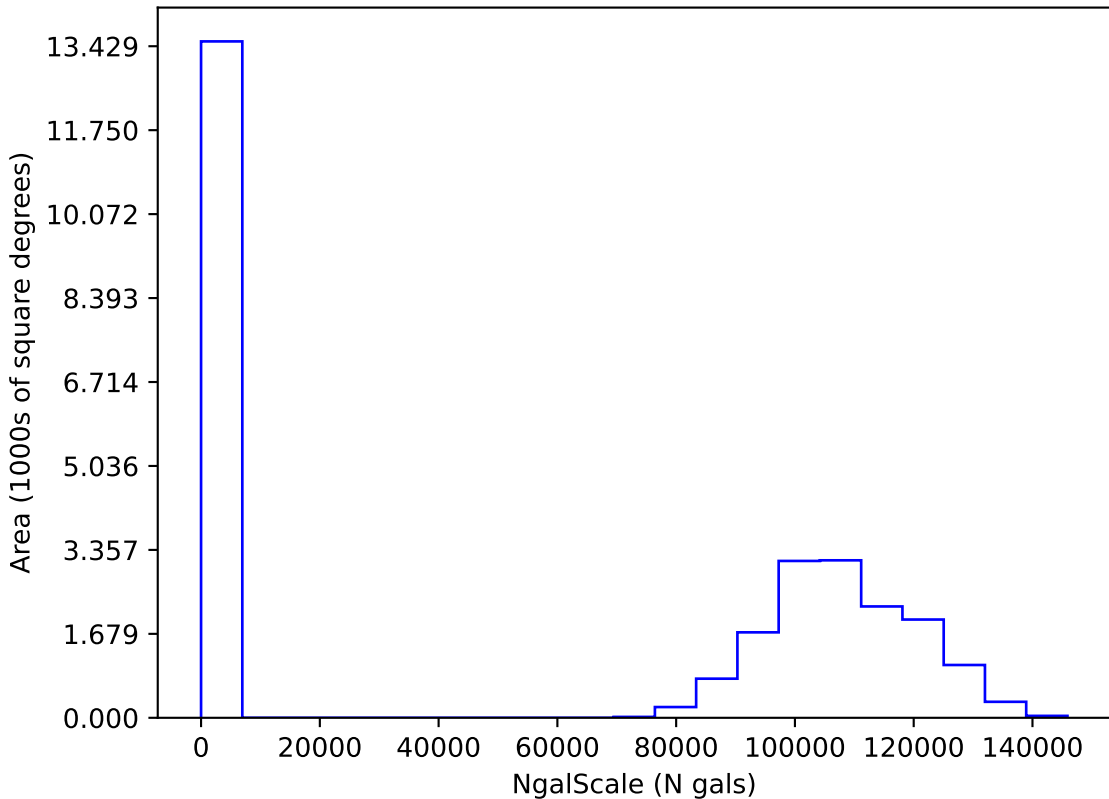
weather_cloudso20v3.4_10yrs i: NgalScale
