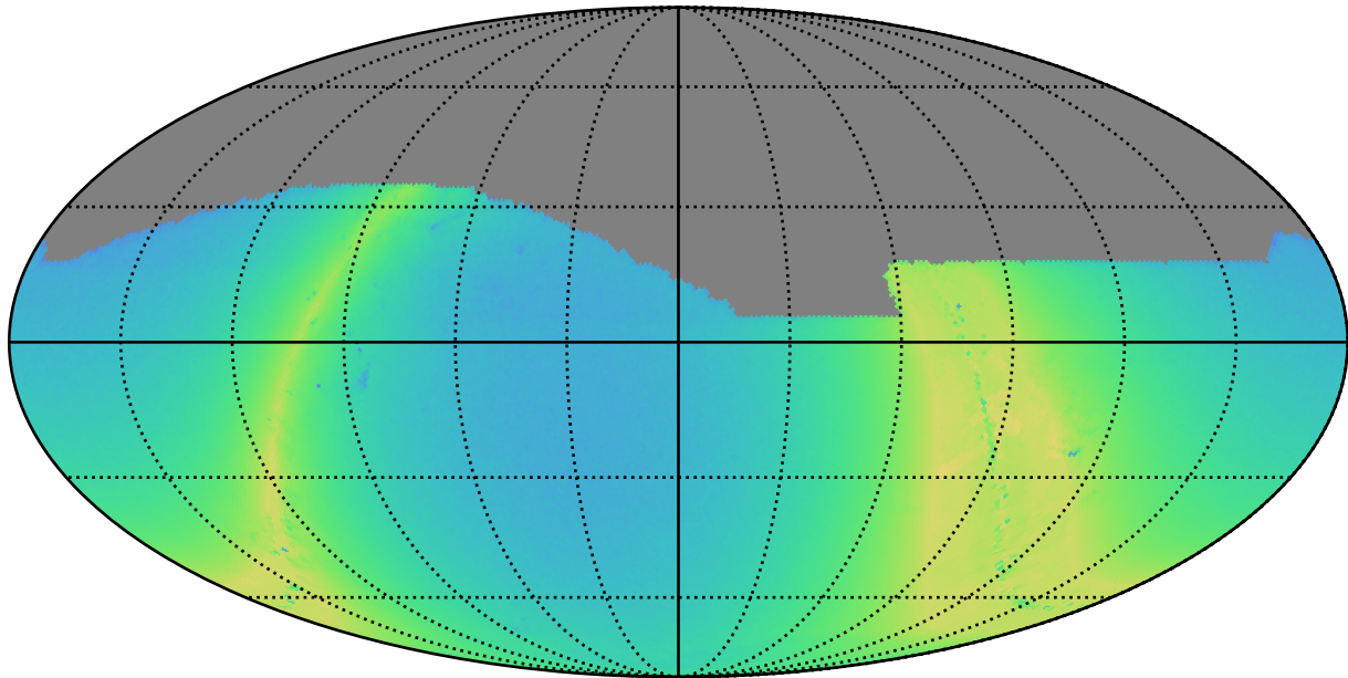
weather_cloudso20v3.4_10yrs i: N stars to Precision 0.20
