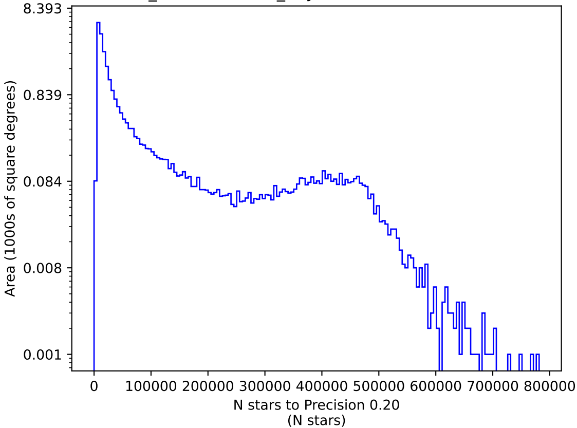
weather_cloudso20v3.4_10yrs i: N stars to Precision 0.20
