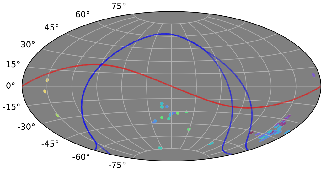
weather_cloudso20v3.4_10yrs gi: LVDwarfs
