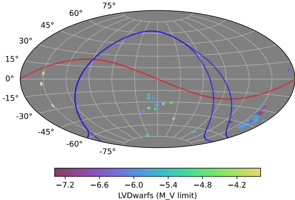
weather_cloudso20v3.4_10yrs gi: LVDwarfs
