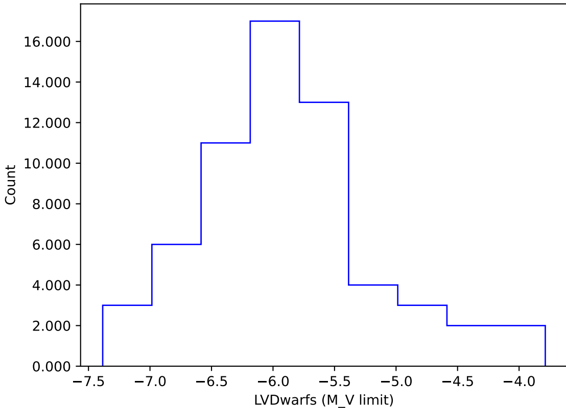
weather_cloudso20v3.4_10yrs gi: LVDwarfs
