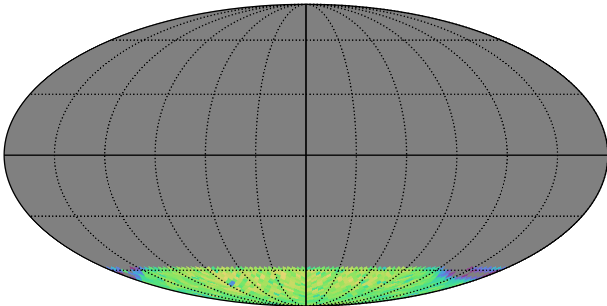
weather_cloudso20v3.4_10yrs gi SCP: LVDwarfs
