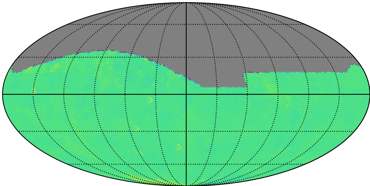
weather_cloudso20v3.4_10yrs z: Kuiper rotTelPos
