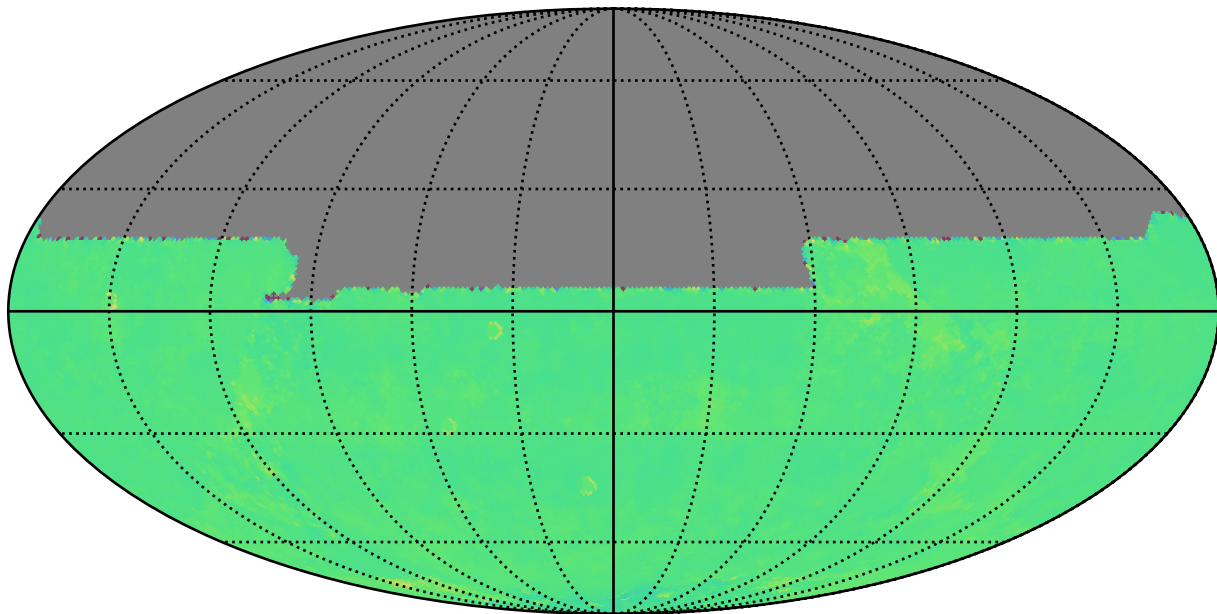
weather_cloudso20v3.4_10yrs y: Kuiper rotTelPos
