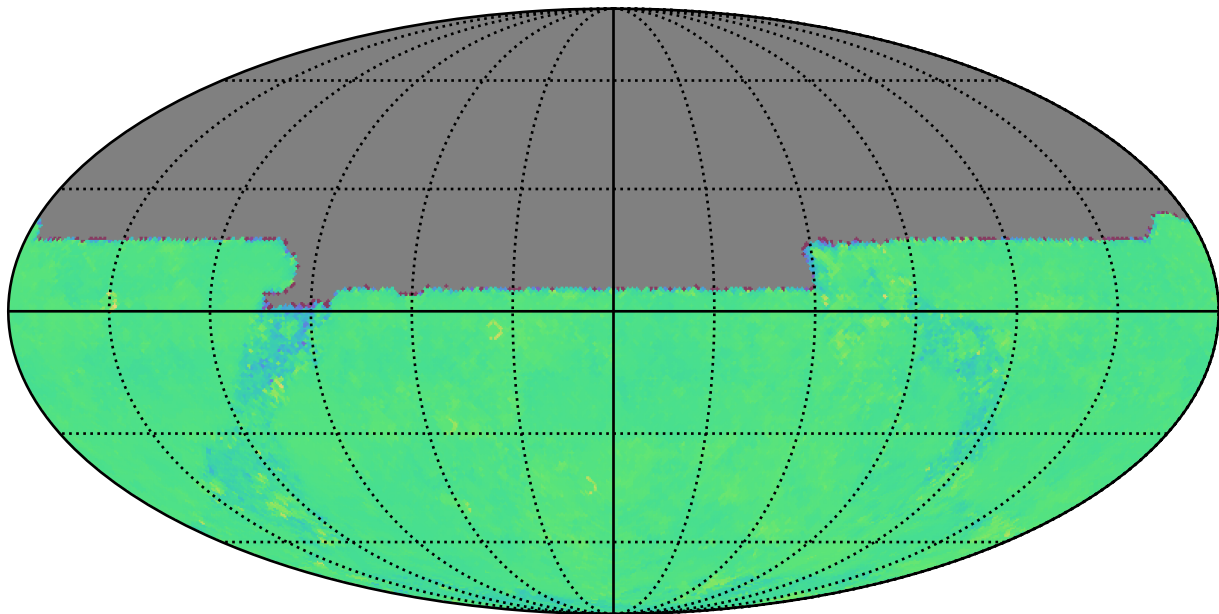
weather_cloudso20v3.4_10yrs u: Kuiper rotTelPos
