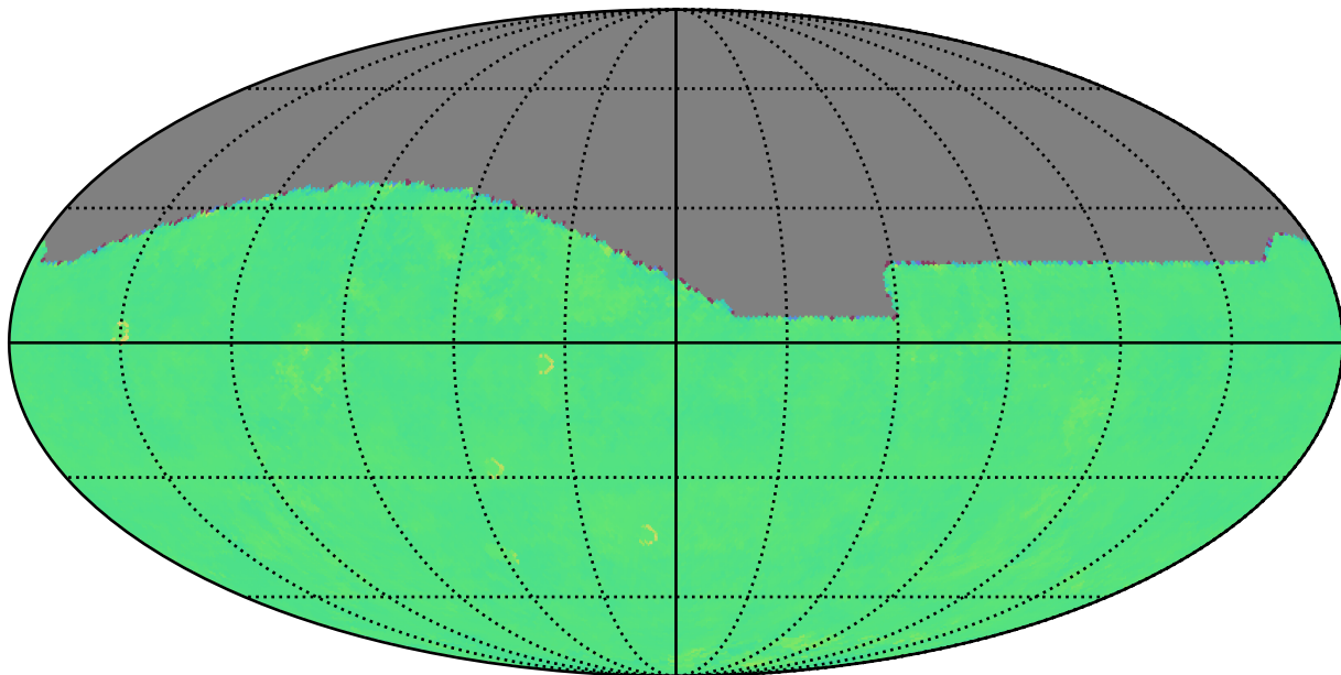
weather_cloudso20v3.4_10yrs r: Kuiper rotTelPos
