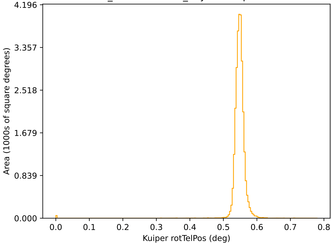
weather_cloudso20v3.4_10yrs r: Kuiper rotTelPos
