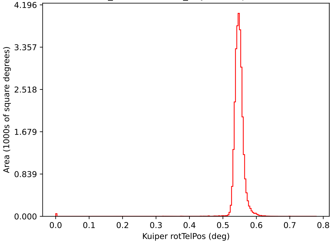
weather_cloudso20v3.4_10yrs i: Kuiper rotTelPos
