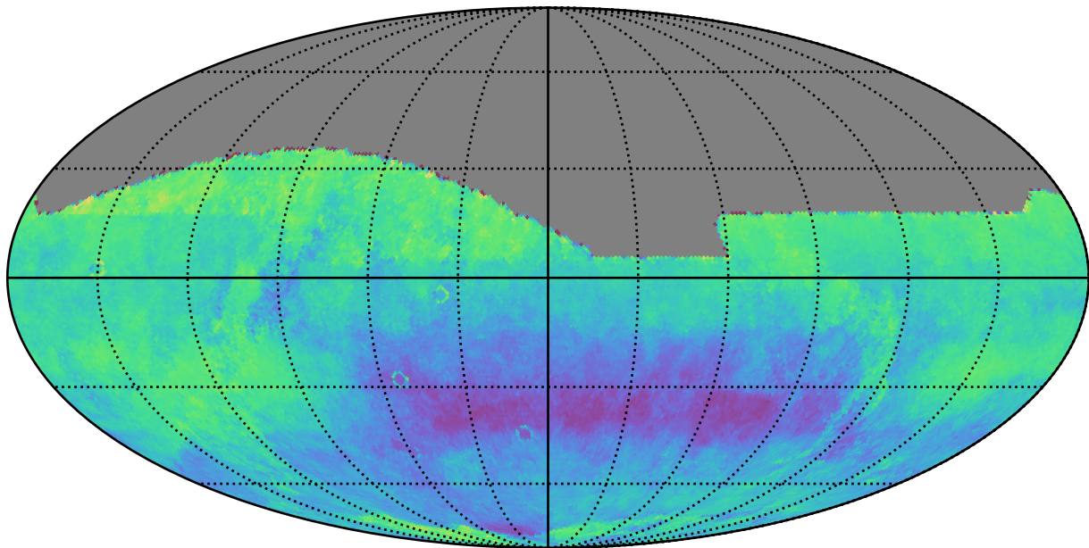
weather_cloudso20v3.4_10yrs z: Kuiper rotSkyPos
