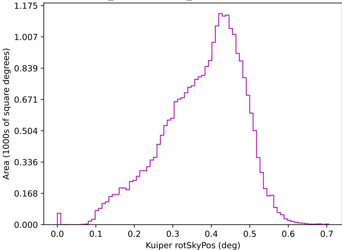
weather_cloudso20v3.4_10yrs z: Kuiper rotSkyPos
