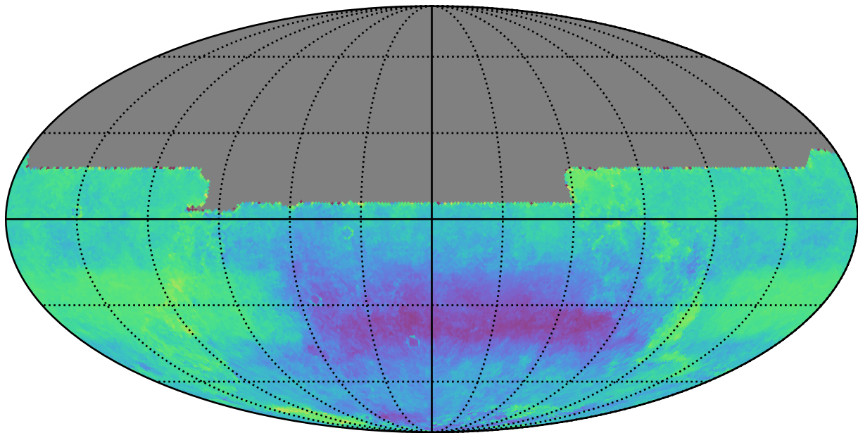
weather_cloudso20v3.4_10yrs y: Kuiper rotSkyPos
