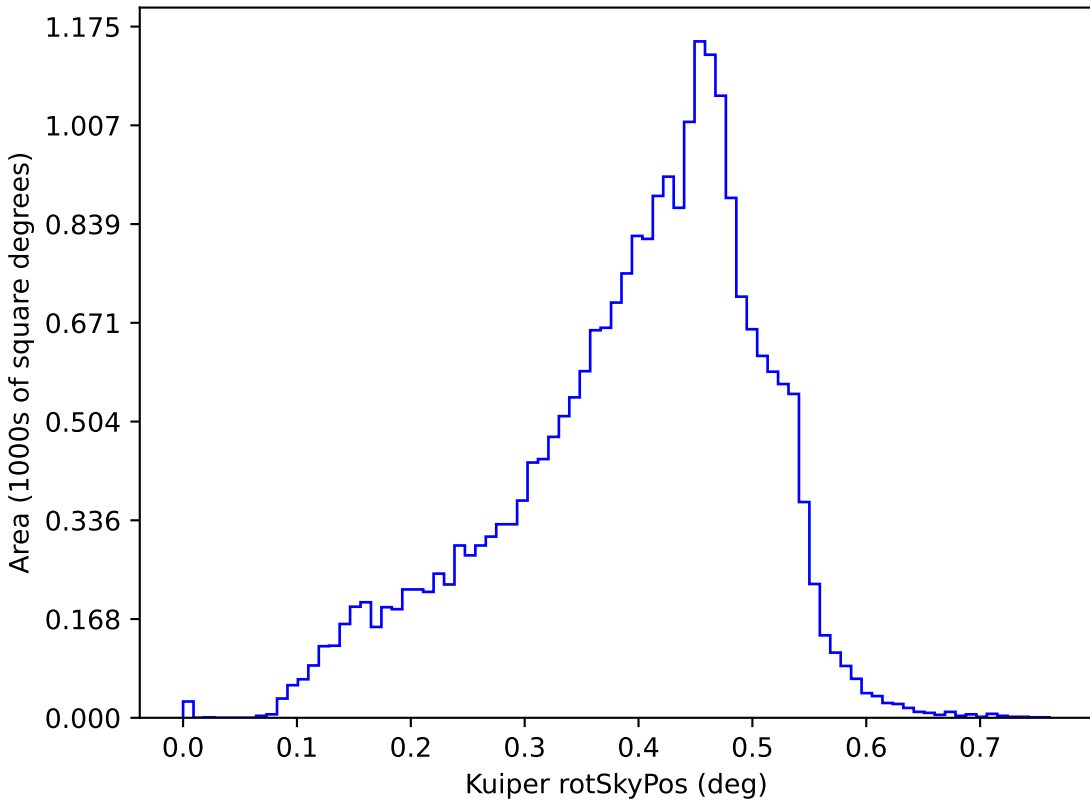
weather_cloudso20v3.4_10yrs y: Kuiper rotSkyPos
