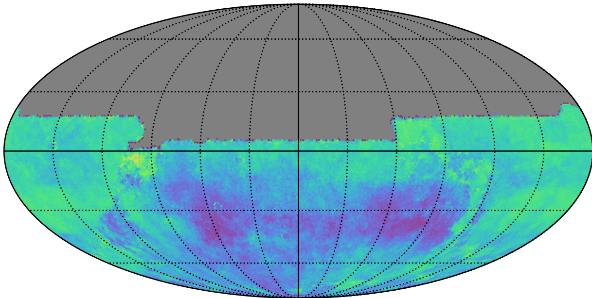
weather_cloudso20v3.4_10yrs u: Kuiper rotSkyPos
