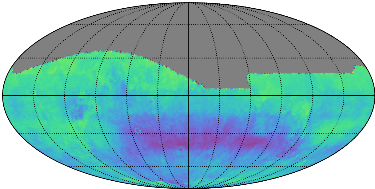
weather_cloudso20v3.4_10yrs i: Kuiper rotSkyPos
