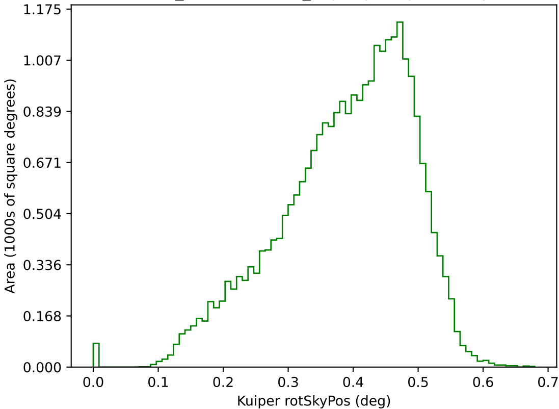
weather_cloudso20v3.4_10yrs g: Kuiper rotSkyPos
