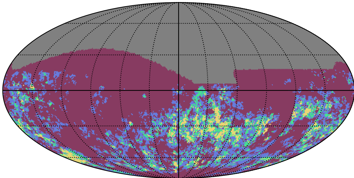
weather_cloudso20v3.4_10yrs z band: Gaps_7hr
